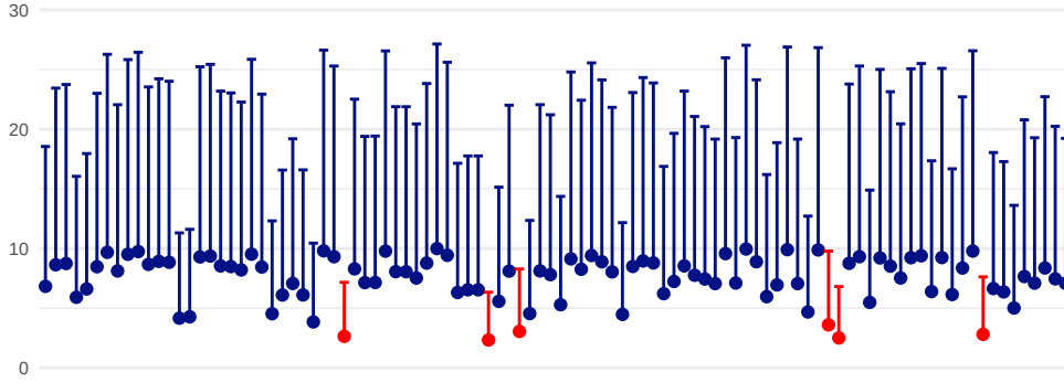
Kuva 8.1: Simuloimalla tuotetuista n = 3 alkion aineistoista väliestimaattorilla \left[\hat{\theta}(\vec{x}), \frac{\hat{\theta}(\vec{x})}{(1-0.95)^{1/3}}\right] laskettuja luottamusvälejä tasajakauman parametrille \theta .
