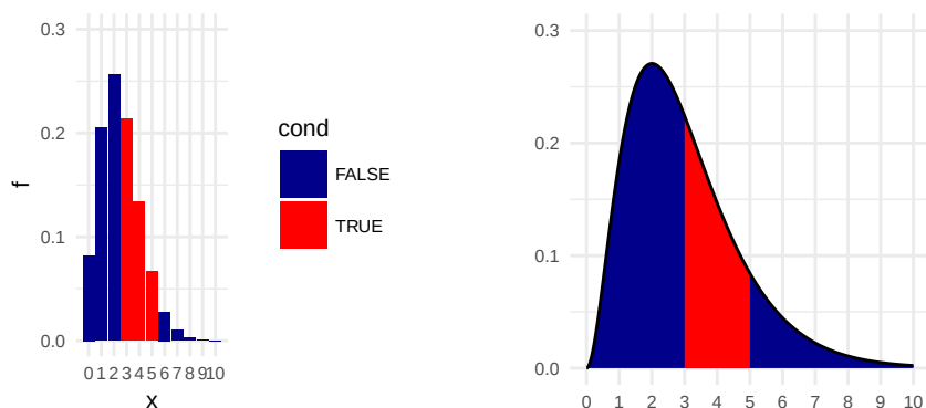
Kuva 2.1: Tapahtuman 3 \leq X \leq 5 todennäköisyys lasketaan diskreetille jakaumalle punaisten pylväiden korkeuksien summana (vasen) ja jatkuvalle jakaumalle punaisen alueen pinta-alana (oikea).
