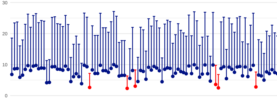
Kuva 8.1: Simuloimalla tuotetuista n = 3 alkion aineistoista väliestimaattorilla \left[\hat{\theta}(\vec{x}), \frac{\hat{\theta}(\vec{x})}{(1-0.95)^{1/3}}\right] laskettuja luottamusvälejä tasajakauman parametrille \theta .
