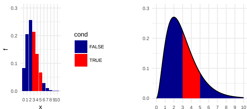
Kuva 2.1: Tapahtuman 3 \leq X \leq 5 todennäköisyys lasketaan diskreetille jakaumalle punaisten pylväiden korkeuksien summana (vasen) ja jatkuvalla jakaumalla punaisen alueen pinta-alana (oikea).
