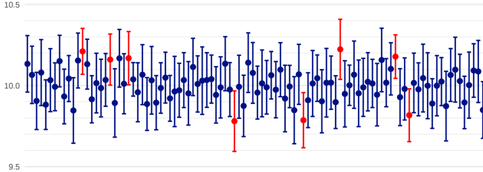
Kuva 8.2: Simuloimalla tuotetuista n = 30 alkion aineistoista väliestimaattorilla m(\vec{x}) \pm 1.96 \frac{\text{sd}(\vec{x})}{\sqrt{n}} laskettuja luottamusvälejä yleisen mallin odotusarvoparametrille \mu .
