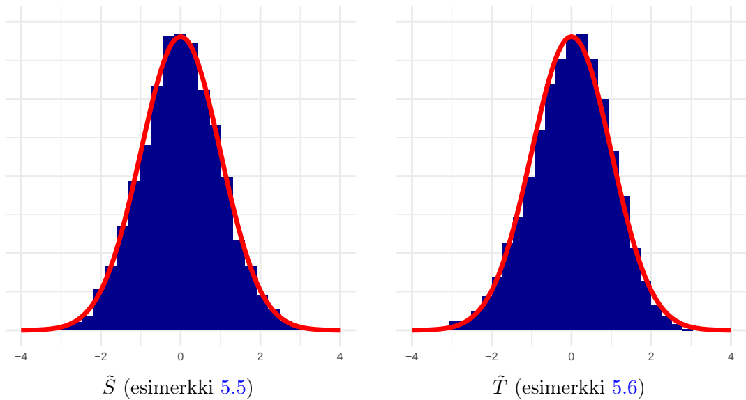
Kuva 5.1: Normitettujen satunnaismuuttujien \tilde{S} ja \tilde{T} simuloidut jakaumat.
